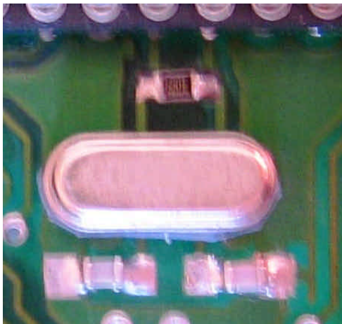
Abbildung 8: Bauteile der die Oszillatorschaltung
