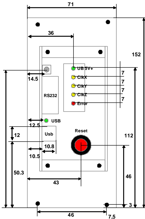
Abbildung 11: Ausgefäste Frontplatte beim Einbau in ein 19“-Gehäuse ohne Kasette
