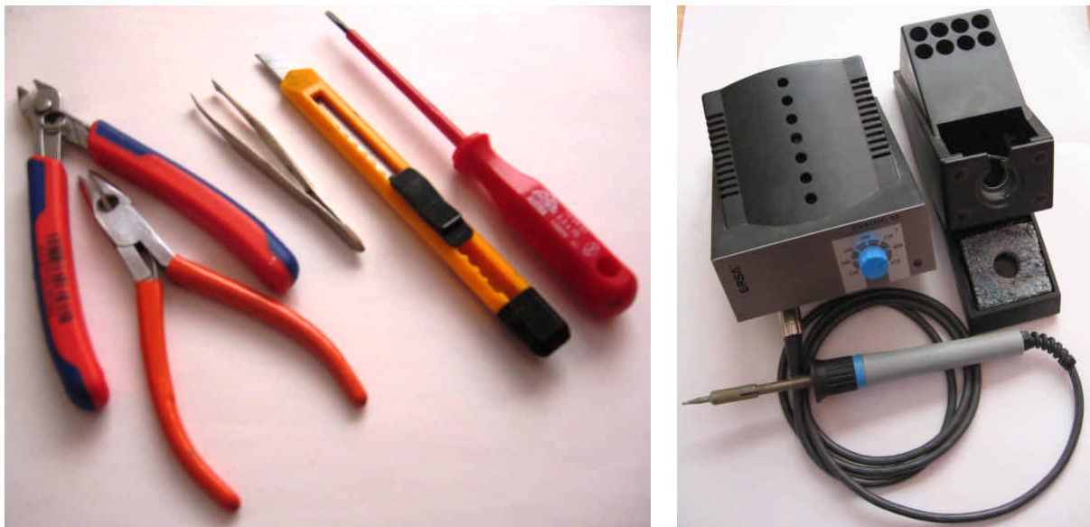
Abbildung 3: Notwendige Werkzeuge zum Aufbau des AKKON USB Controller Board
