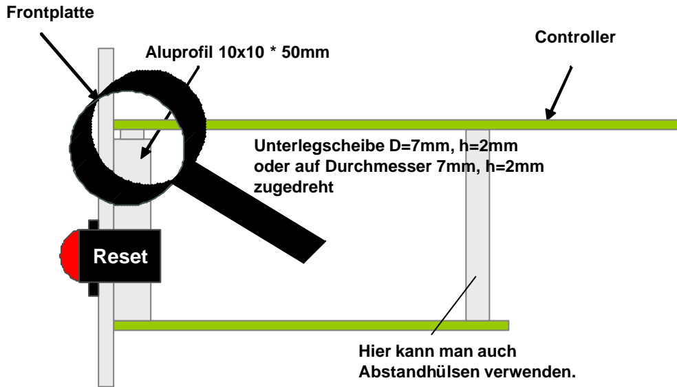
Abbildung 12: Alternative Befestigungsmöglichkeit wenn keine 19" Kasette verwendet wird
