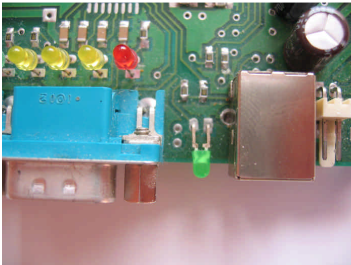
Abbildung 10: Richtiger Einbau der Leuchtdioden
