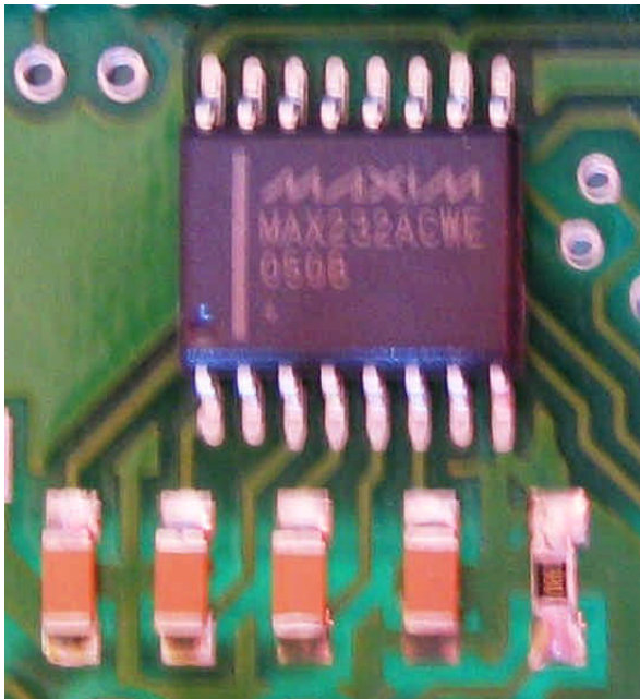
Abbildung 7: Ansicht der Bauteile für die RS232-Schnittstelle
